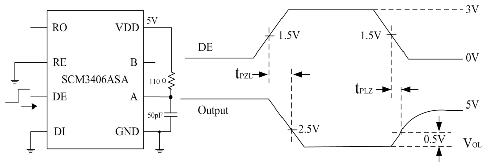
图 21 驱动器使能/禁能测试电路及波形，低电平输出
