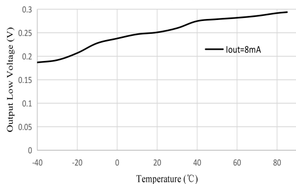
图5 接收器输出低电压 VS 温度
