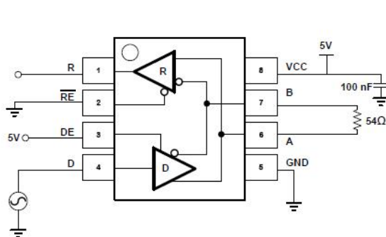
图15 回环测试及其波形
