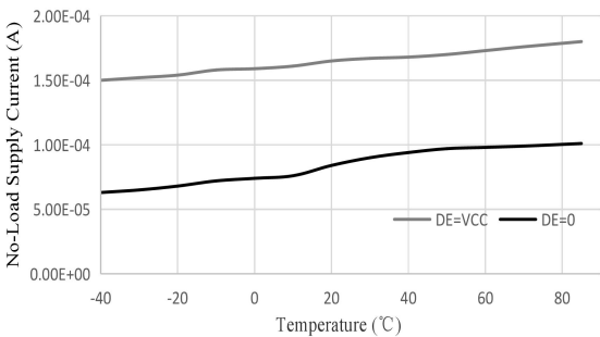
图 1 供电电流（空载） VS. 温度
