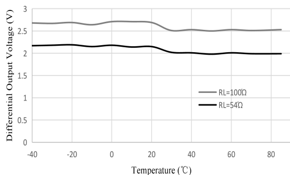
图7 驱动器差分输出电压 VS 温度
