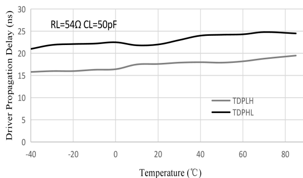
图14 驱动器传输延时 VS 温度
