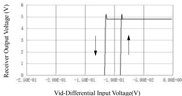
图12 接收器输出电压 VS 差分输入电压
